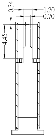
剖視圖
