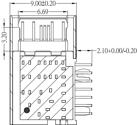
剖視圖
